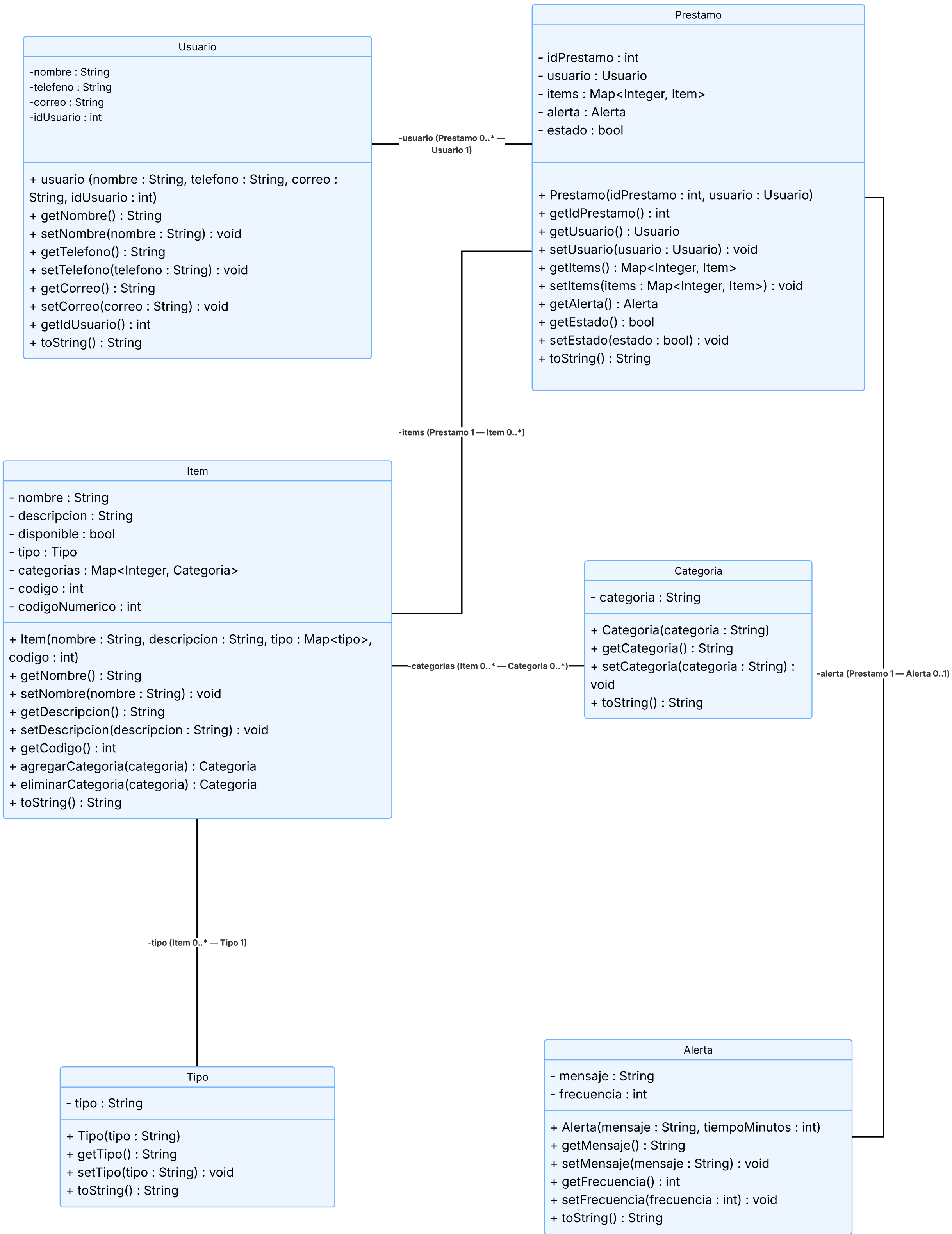
Lógica: Diagrama de Clases
